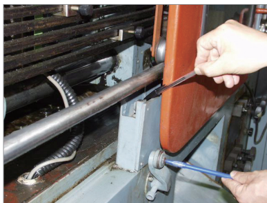
전기식(리미트 스위치) 설치
