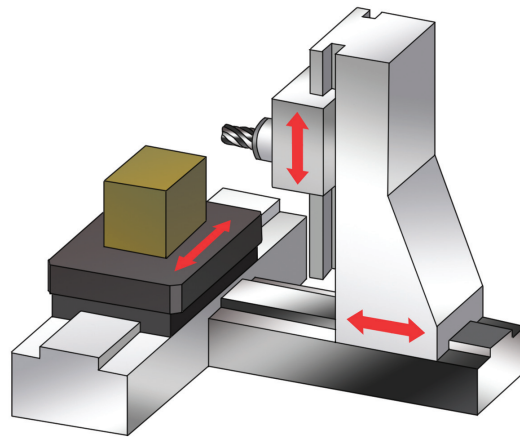
수평형 머시닝 센터
